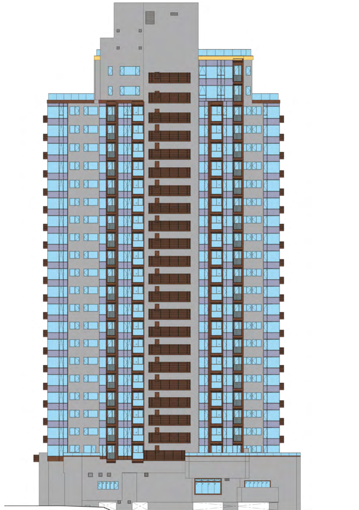
立面圖 1 Elevation 1
